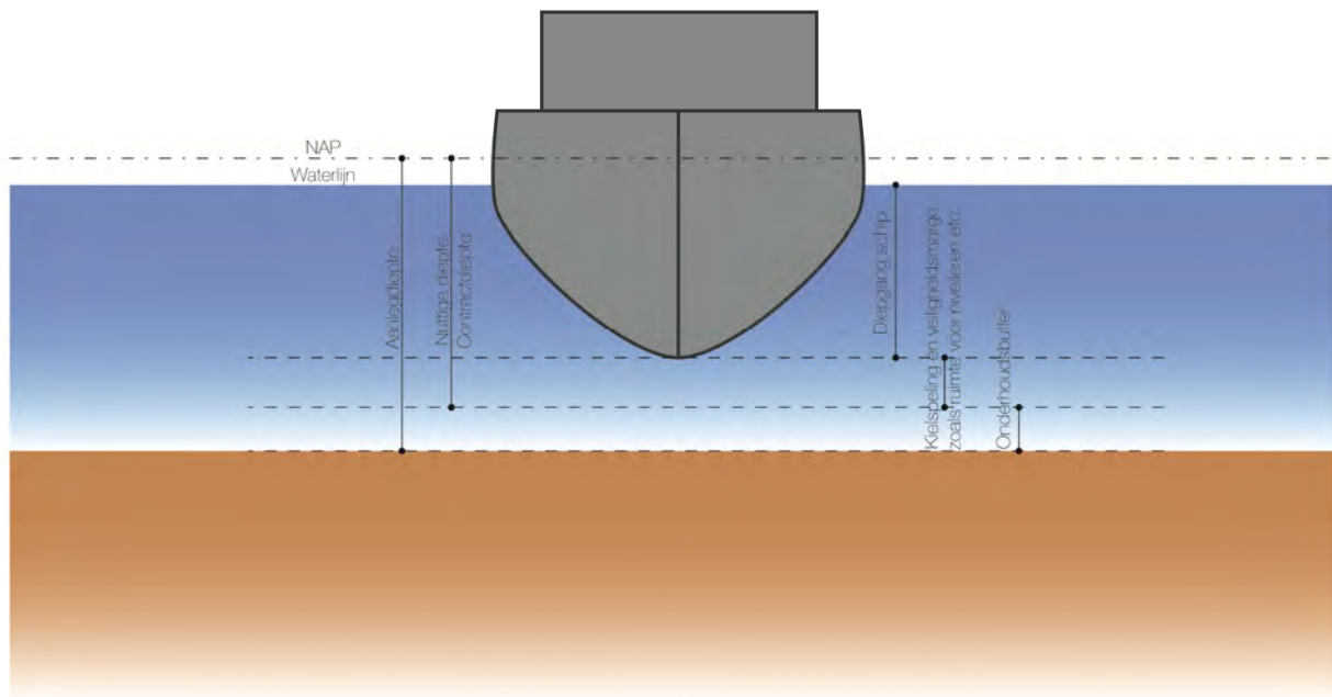
Figuur 0-1: Nuttige diepte, contractdiepte, aanlegdiepte.
