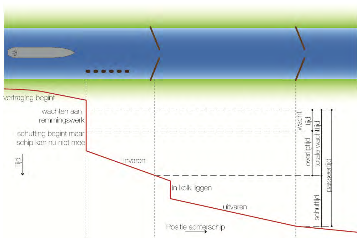
Figuur 0-2 Passeertijd = totale wachttijd + schuttijd. Totale wachttijd = wachttijd + overligtijd.
